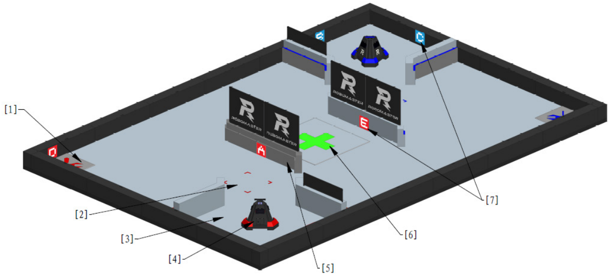
图 5-4 3V3 对抗赛木质场地轴测图
