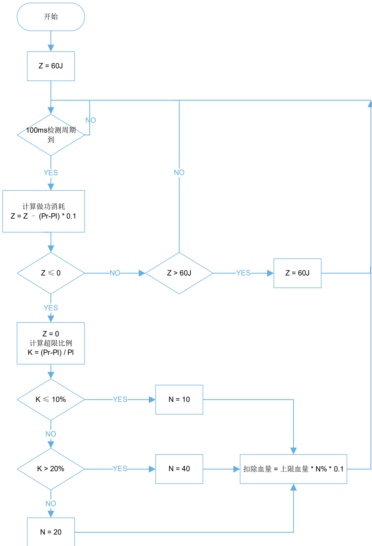
图 4-4 步兵机器人和英雄机器人底盘功率检测及扣血逻辑图
