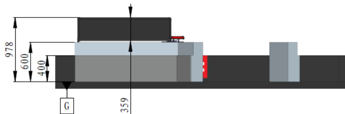
图 5-8 木质场地启动区示意图
