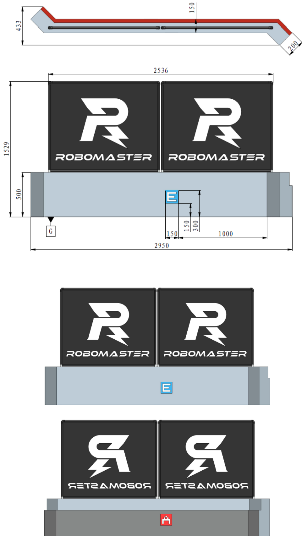
图 5-11 木质场地掩体示意图
