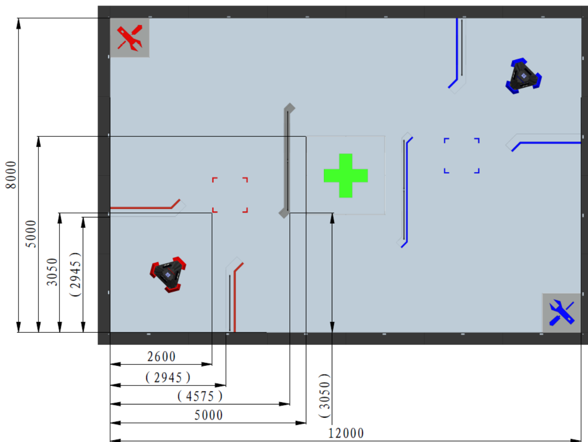
图 5-6 3V3 对抗赛木质场地尺寸示意图
