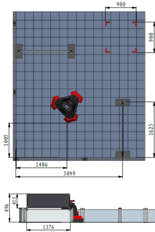
图 5-7 拼接场地启动区示意图
