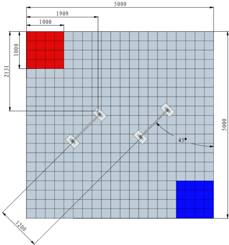
图 5-21 步兵对抗赛拼接场地尺寸示意图
