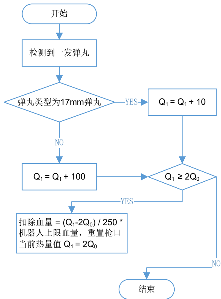
图 4-2 枪口热量超限的扣血逻辑图
