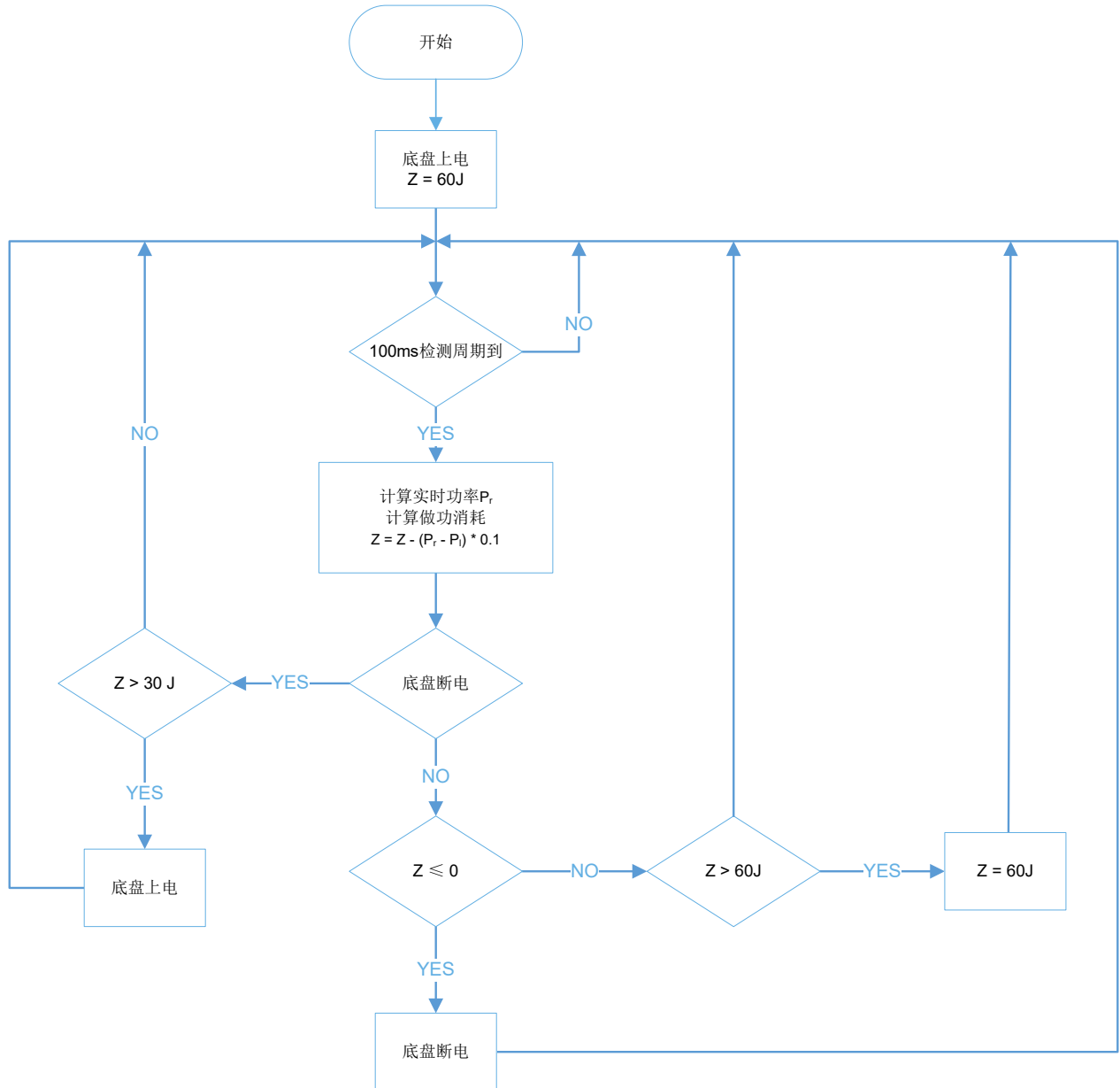
图 4-5 哨兵机器人底盘功率检测及底盘断电逻辑图
