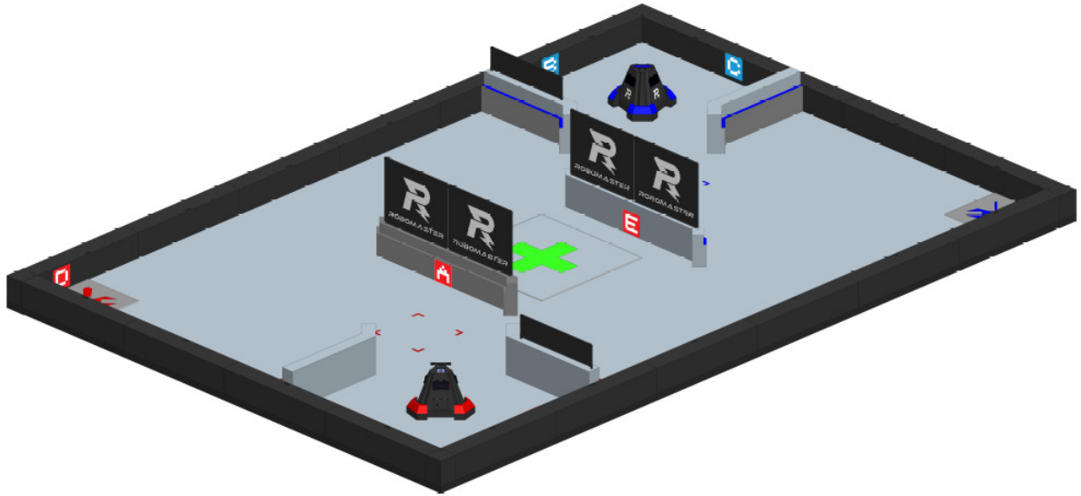
图 5-4 3V3 对抗赛木质场地轴测图
