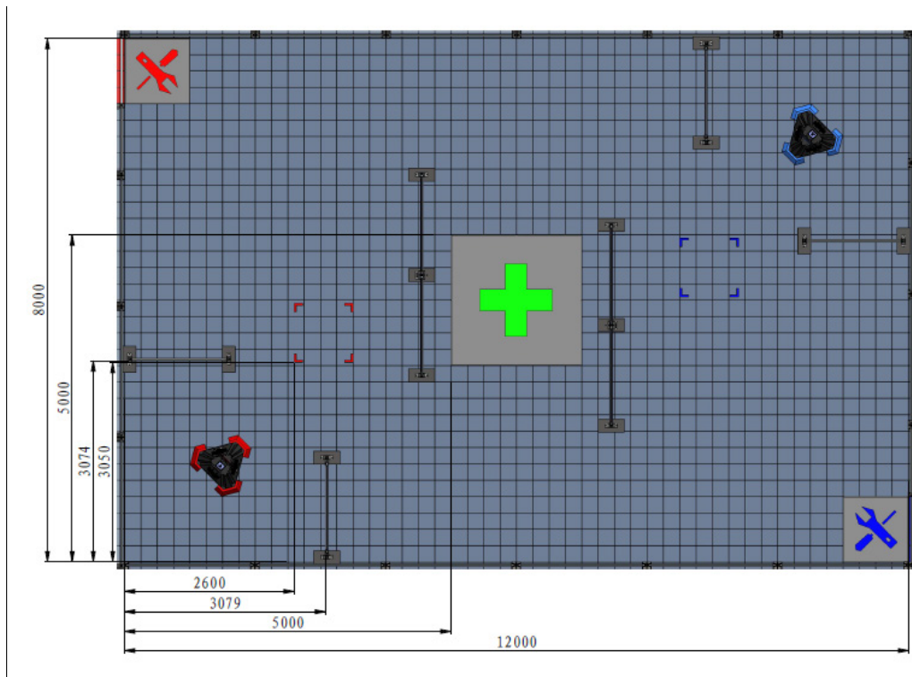
图 5-3 3V3 对抗赛拼接场地尺寸示意图
